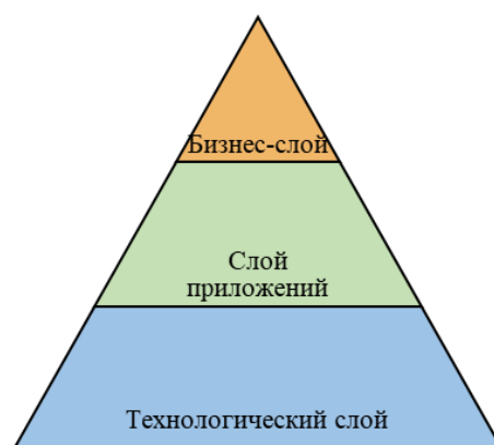
Рис. 3. Домены TOGAF
