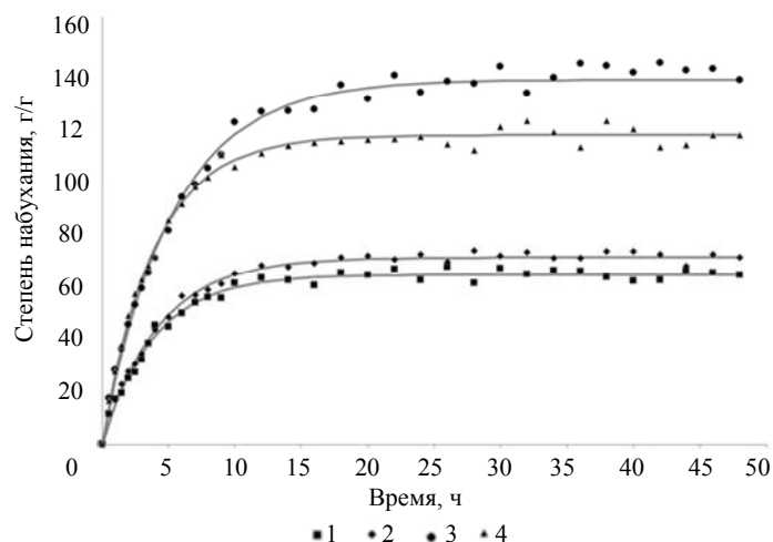
Рис. 1. Кинетические кривые набухания акрилового композита, модифицированного частицами бентонита с массовой долей 2 мас. % при температуре 20°C в дистиллированной воде: 1 – акриловый гидрогель без наполнителя; 2 – гидрогель, модифицированный натриевым бентонитом; 3 – гидрогель, модифицированный Ag-содержащим бентонитом с дисперсностью частиц d < 0,25 мм; 4 – гидрогель, модифицированный Ag-содержащим бентонитом с дисперсностью частиц d = 0,25 - 0,5 мм
