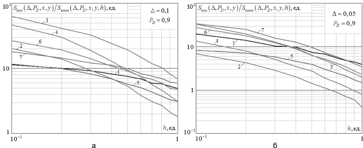
Рис. 5. Оценка эффективности критерия программной компенсации технологического разброса (x,y) -координат цветности: \Delta=0,1 (а); \Delta=0,05 для метода, основанного на измерении координат XYZ (б). 1 – белый RGB=(250,250,250) ; 2 – красный RGB=(250,10,10) ; 3 – зеленый RGB=(10,250,10) ; 4 – синий RGB=(10,10,250) ; 5 – желтый RGB=(250,250,10) ; 6 – пурпурный RGB=(250,10,250) ; 7 – голубой RGB=(10,250,250)
