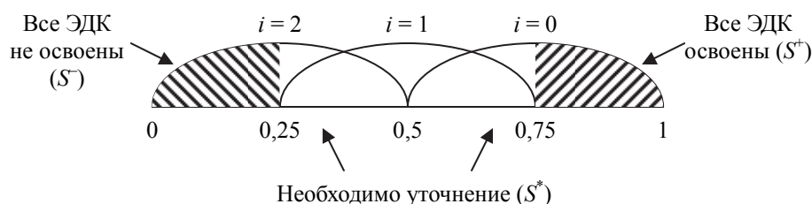
Рис. 1. Графическая иллюстрация анализа результатов тестирования для h = 2
