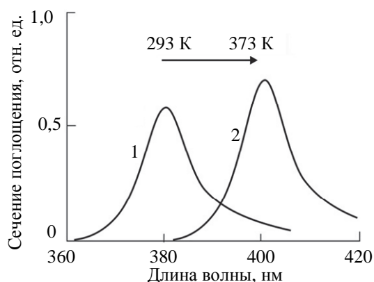
Рис. 2. Расчетные спектры сечения поглощения наночастиц натрия в стекле в твердой (1) и жидкой (2) фазах
