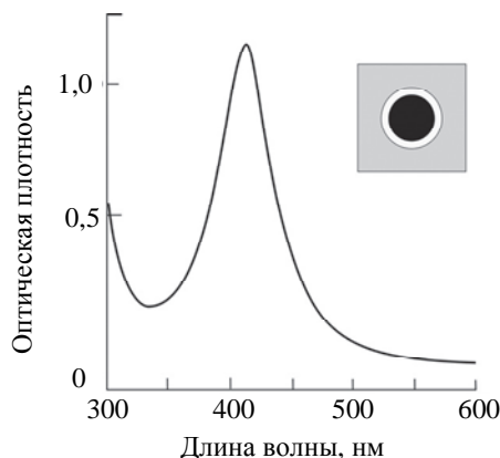
Рис. 1. Спектр оптической плотности силикатного стекла с наночастицами натрия. На вставке – геометрия наночастицы
