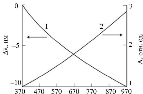
Рис. 4. Температурные зависимости спектрального сдвига ( \Delta\lambda ) и амплитуды ( A ) максимума плазмонной полосы поглощения наночастиц натрия в жидкой фазе
