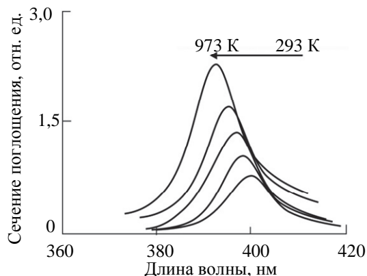
Рис. 3. Расчетные спектры сечения поглощения наночастиц натрия в стекле в жидкой фазе в температурном интервале 373–973 К
