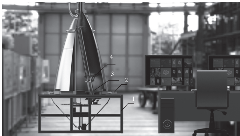
Рис. 5. Общий вид макета автоматизированной лазерно-ультразвуковой установки неразрушающего контроля: 1 – каркасное основание; 2 – устройство центрирование объекта контроля; 3 – устройство позиционирования; 4 – устройство обеспечения акустического контакта
