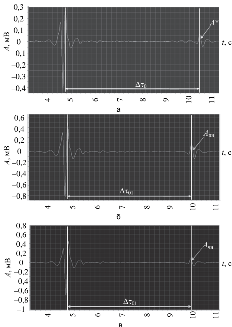
Рис. 4. Вид А-сканов при ультразвуковом контроле: бездефектное паяное соединение (а); полный непропай (б); частичный непропай (в). A – амплитуда сигнала, мВ; A^* – амплитуда донного сигнала, мВ; A_{чн} – амплитуда сигнала, отраженного от границы раздела сред при частичном непропае, мВ; A_{пн} – амплитуда сигнала, отраженного от границы раздела сред при полном непропае, мВ; t – время прохождения сигнала, с; \Delta\tau_0 – время между зондирующим ультразвуковым сигналом и первым отраженным ультразвуковым сигналом, с; \Delta\tau_{01} – время между зондирующим ультразвуковым сигналом и первым отраженным от дефекта ультразвуковым сигналом, с
