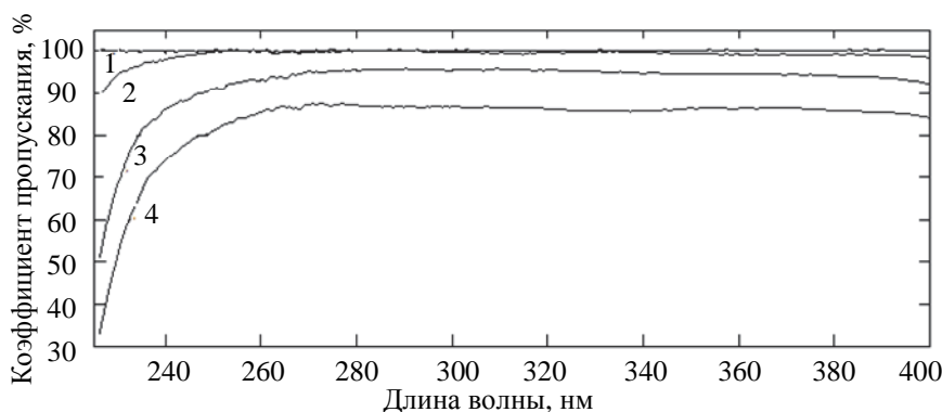
Рис. 3. Измеренные экспериментально спектры ультрафиолетового коэффициента пропускания T(\lambda) водных растворов карбамида. Концентрация раствора m_d , %: 1 – 0; 2 – 15; 3 – 30; 4 – 50
