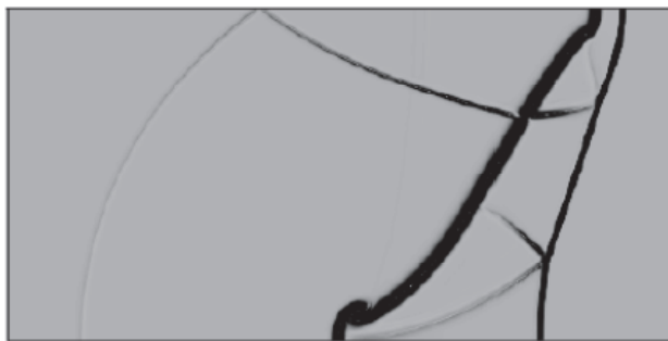
Рис. 5. Численная теньевая картина
