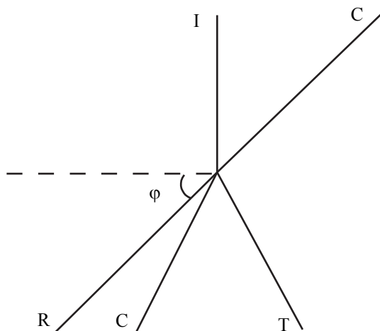
Рис. 1. Рефракция ударной волны на контактном разрыве
