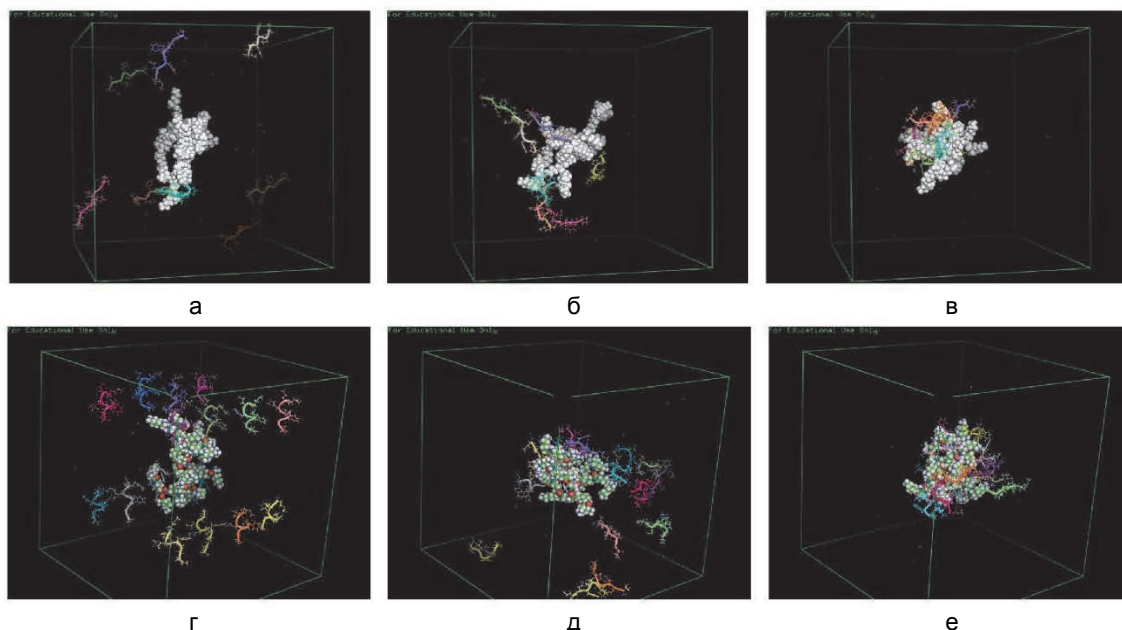
Рис. 2. Стадии формирования комплекса дендримера (начальная, промежуточная и конечная) и пептидов Семакс: система дендример и 8 пептидов: t = 0 (а); t = 20 нс (б); t = 160 нс (в); система дендример и 16 пептидов: t = 0 (г); t = 20 нс; (д); t = 160 нс (е). Атомы молекулы дендримера (в центре) на рисунке показаны шариками с диаметрами, равными их ван-дер-ваальсовым радиусам. Валентные связи различных пептидов изображены на рисунке цветными линиями разного цвета
