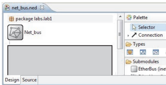
Рис. 2. Окно графического редактора NED-файлов с двумя вкладками
