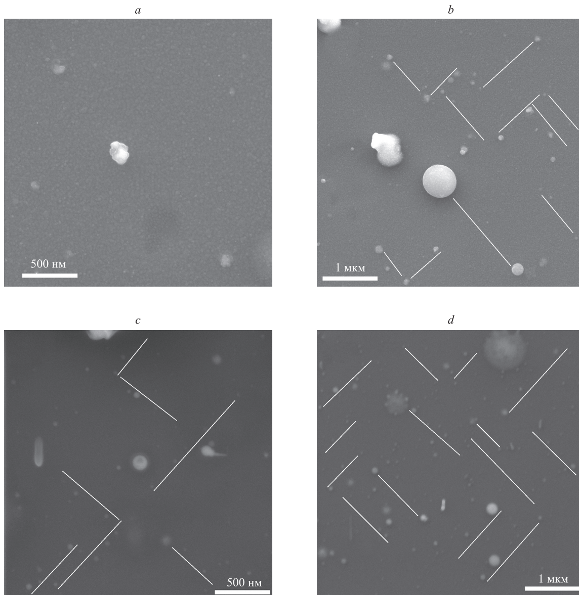
Рис. 2. СЭМ-изображения поверхности тонкой пленки InGaAsN на GaAs (a) и кремниевой (b) подложках и микрокапель индия (c, d)
