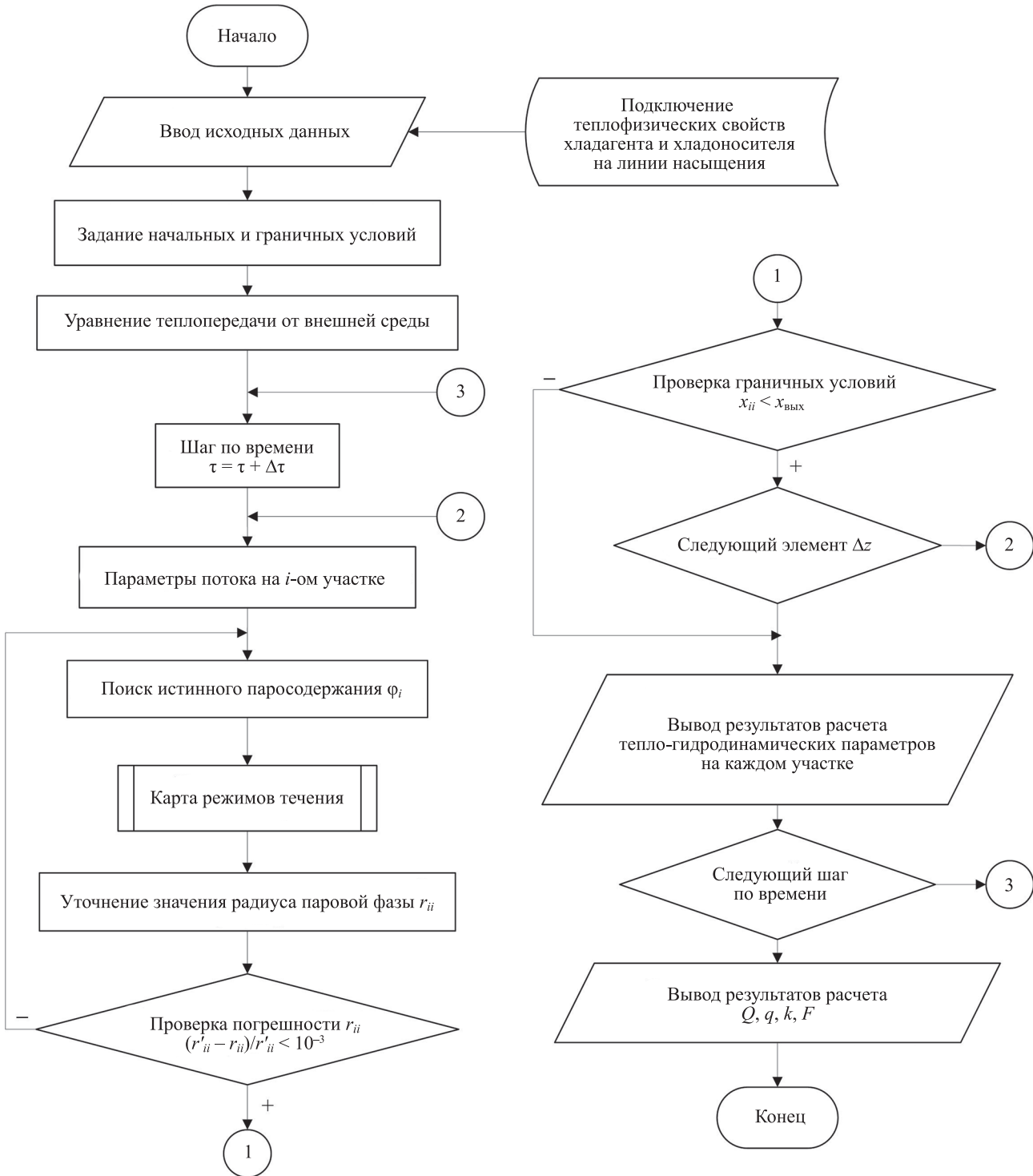
Рис. 2. Обобщенная блок-схема модели расчета процессов кипения в канале Fig. 2. Generalized block diagram of the model for calculating boiling processes in a channel
