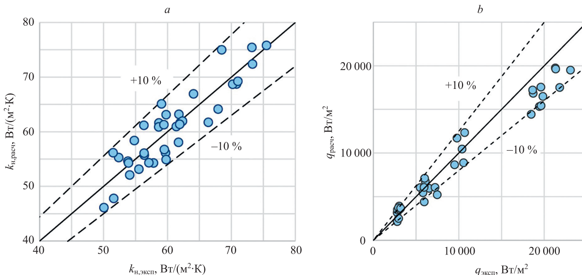
Рис. 3. Результаты сопоставления данных расчетов и экспериментов при кипении: R410a в трубах охлаждающей батареи с микро-оребрением (а) и R22 в гофрированном щелевом канале (b)
