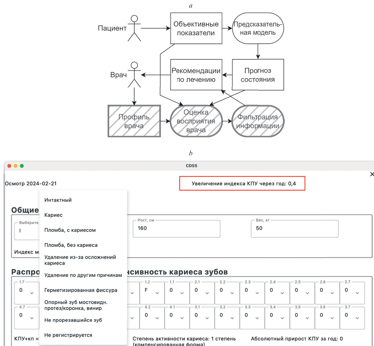
Рисунок. Реализация системы поддержки принятия врачебных решений (СППВР) с оценкой восприятия врача: общая схема расширения СППВР (a); прототип СППВР в рамках профилактического приема врача-стоматолога (b)
