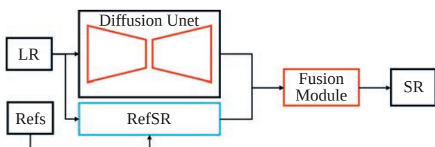
Рис. 1. Предложенная гибридная модель восстановления изображения.
