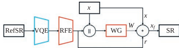
Рис. 2. Схема предложенного модуля слияния (Fusion Module).
