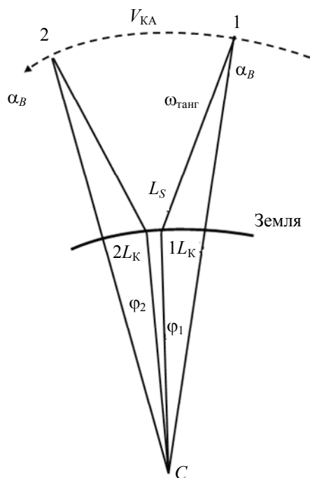
Рис. 3. Плоскость орбиты
