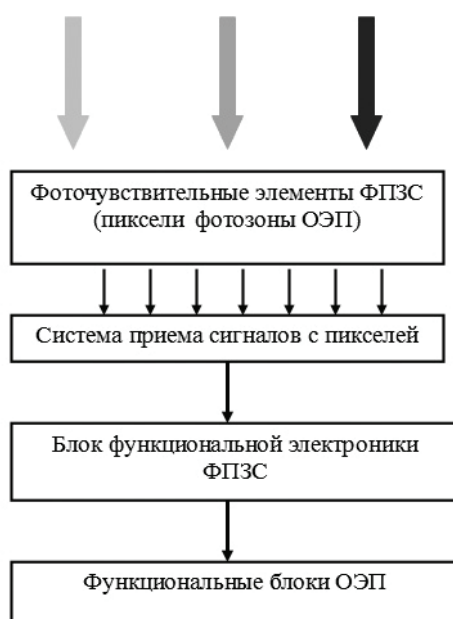
Рис. 2. Обобщенная структурная схема оптико-электронного преобразователя ОЭК ДЗЗ
