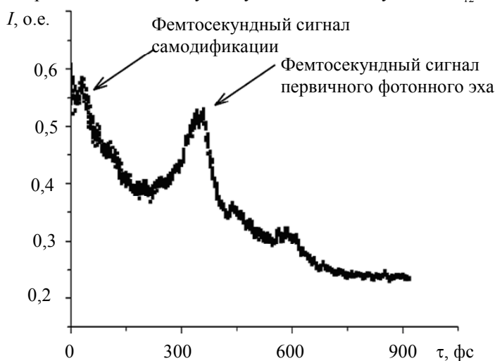
Рис. 2. Интенсивность спада фемтосекундного сигнала самодифракции и фотонного эха при различной разности хода между возбуждающими импульсами
