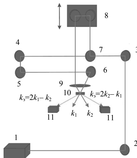
Рис. 1. Оптическая схема фемтосекундного эхо-спектрометра: 1 – фемтосекундная лазерная система; 2–6 – зеркала; 7 – диэлектрический светоделитель; 8 – оптическая линия задержки; 9 – линза; 10 – объект исследования; 11 – фотодетектор, спектрометр. k_1 – волновой вектор первого возбуждающего импульса; k_2 – волновой вектор второго возбуждающего импульса
