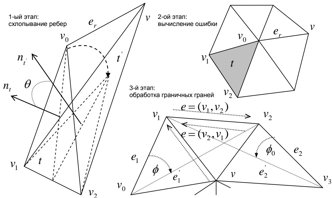
Рис. 2. Свертывание ребер
