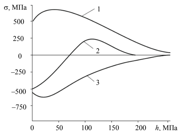
Рис. 2. Распределение остаточных напряжений \sigma(h) в стали 20X13 после обработки: 1 – ручное шлифование на станке ЛШ-95 (Германия); 2 – шлифование лентой на станке Metabo (Германия); 3 – фрезерование на станке Forest (Германия)
