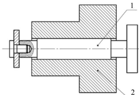
Рис. 3. Схема перемещения штока (1) во втулке (2) в запорном клапане
