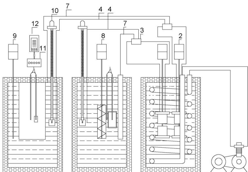
Рисунок – Схема установки для определения ТФХ пищевых продуктов
