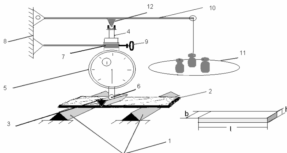
Рис.1 Схема экспериментальной установки по определению хрупкости вафель
