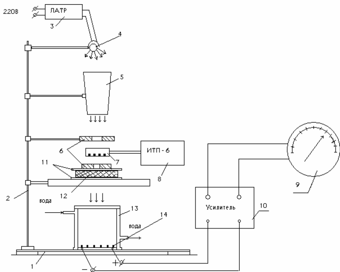
Рис. 1 Установка для определения оптической прозрачности пищевых материалов (коэффициент пропускания).
