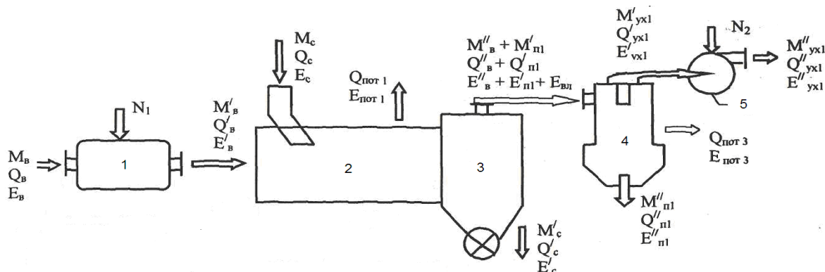
Рис. 1. Схема материального, теплового и эксергетического потоков в барабанном сушильном агрегате
